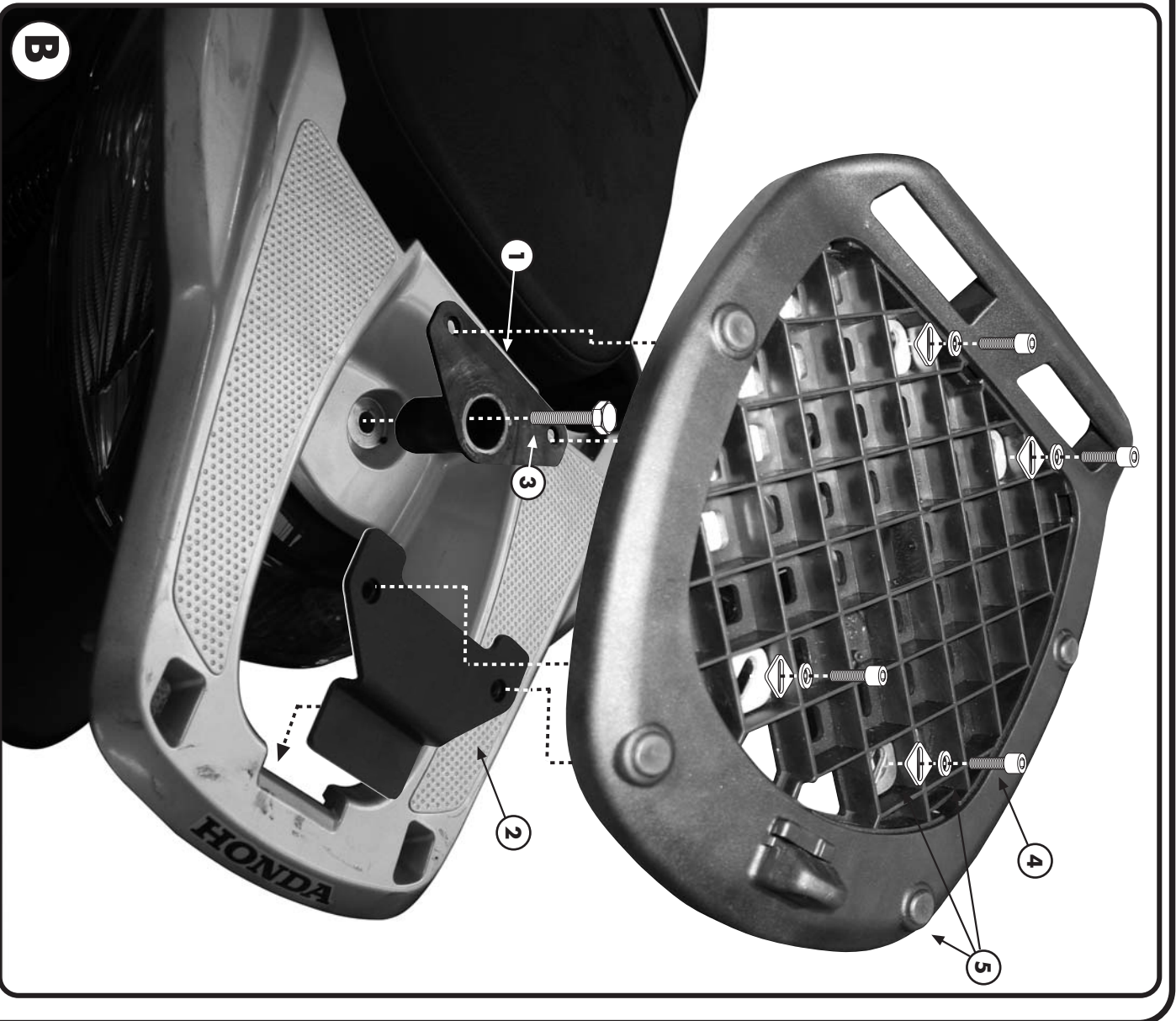
4 VITE TCEI M6x20mm SCREW M6x20mm VIS M6x20mm SCHRAUBE M6x20mm TORNILLO M6x20mm Q.TY n.4
